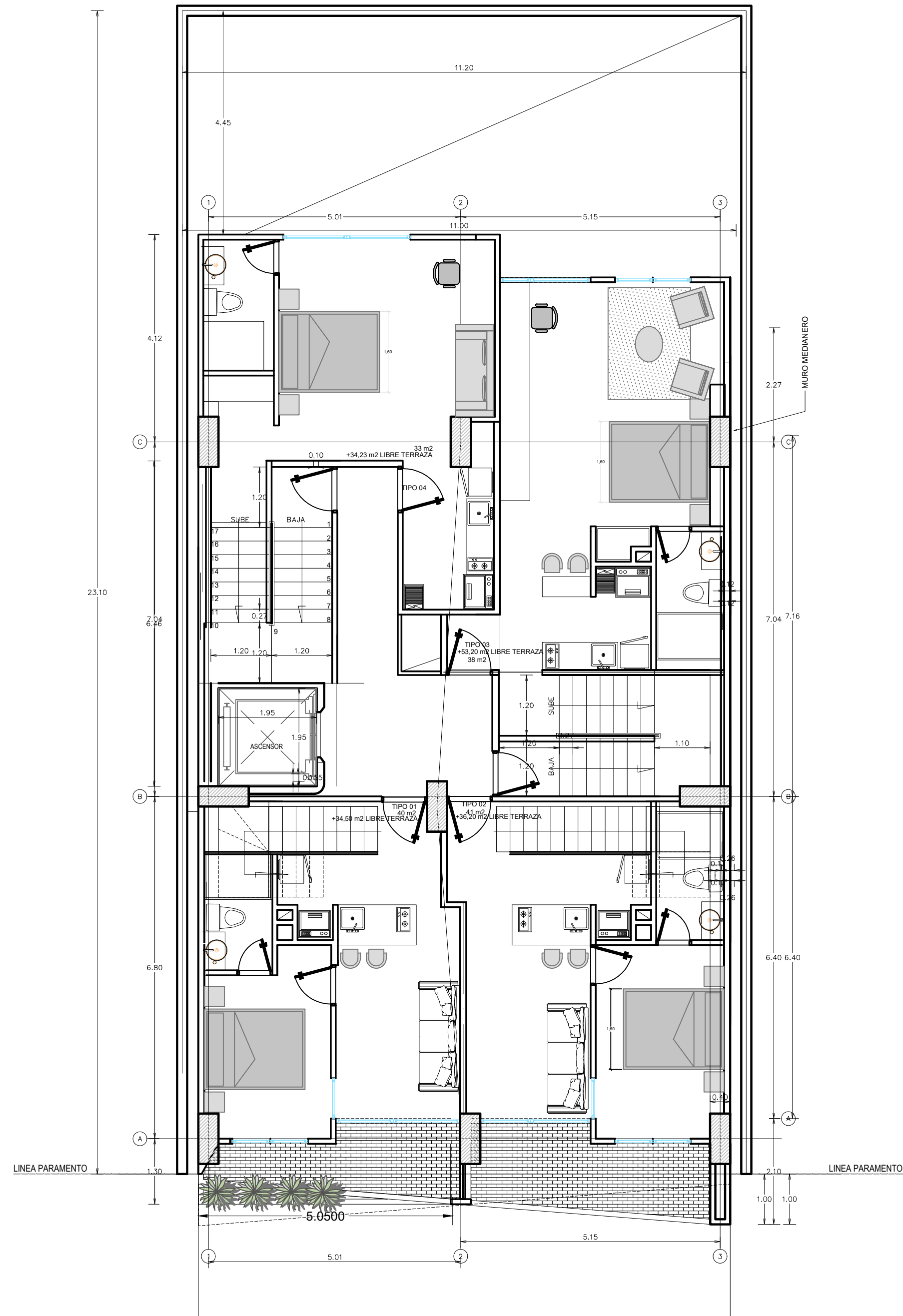
PISO 12
